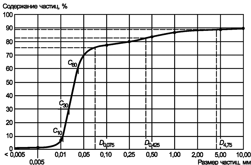
Рисунок Е.2 - Кумулятивная кривая гранулометрического состава
