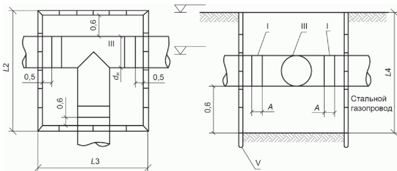
Рисунок А.2 - Установка тройника в монтажном котловане
