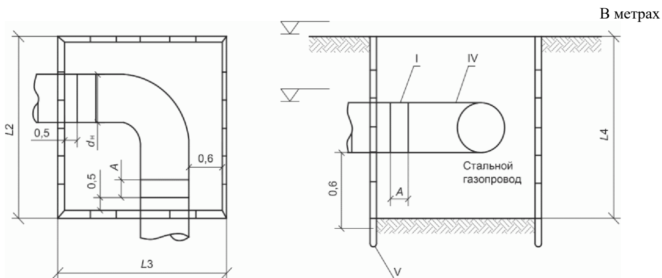
Рисунок А.3 - Установка отвода в монтажном котловане
